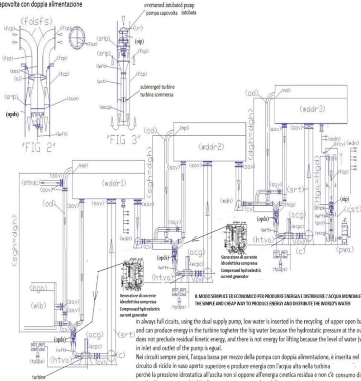
Sistema di sollevamento idroelettrico a gradini sommerso rinforzato con sistema idroelettrico compresso Reinforced submersed stepped hydroelectric lift system with compressed hydroelectric system
